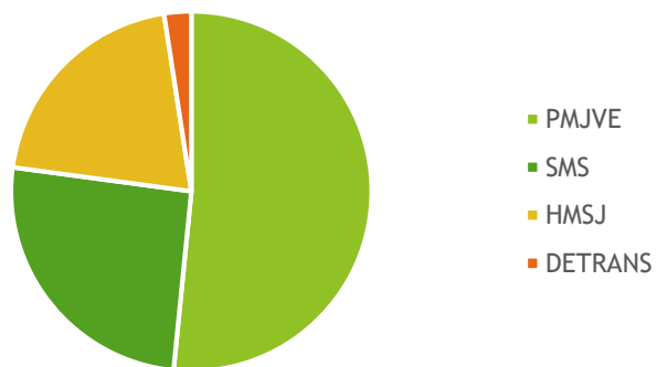
Quantidade Licitações por Instituição
