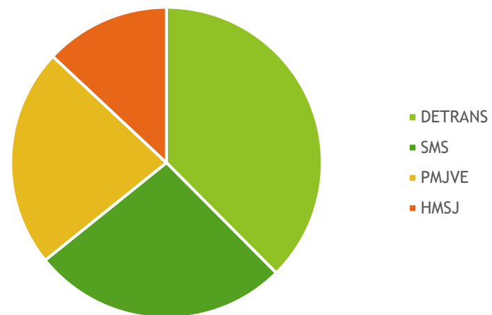
Valor Licitações por Instituição
